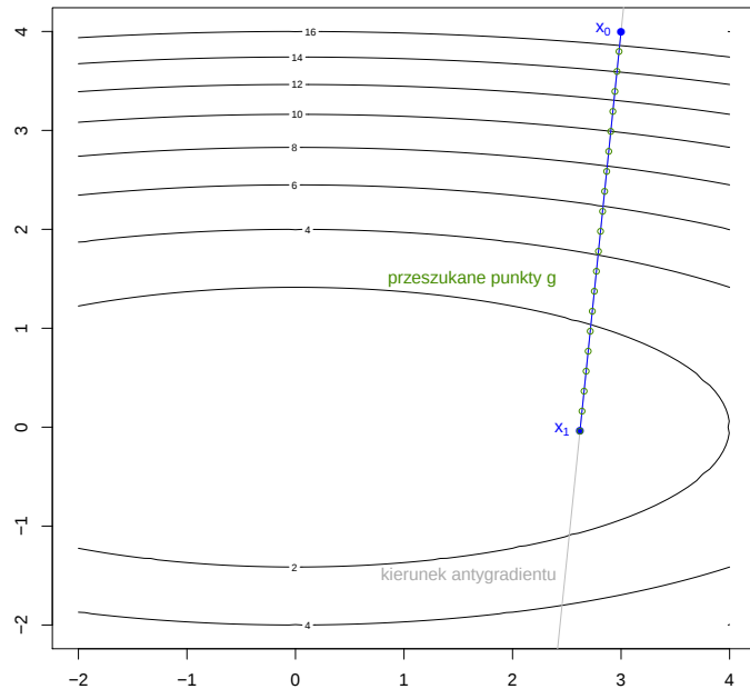
Figure 4.19: Punkty badane podczas jednej iteracji metody najszybszego spadku na funkcji f
