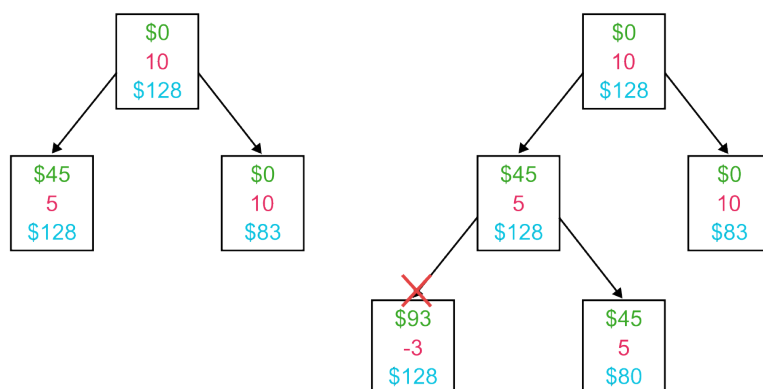
Figure 8.35: Rozszerzanie drzewa 1
