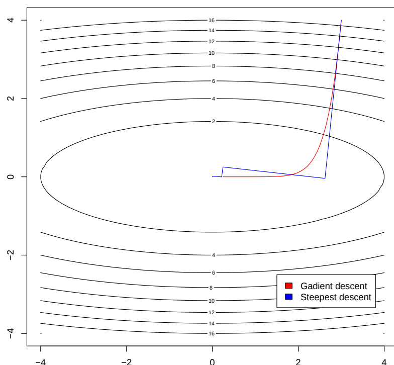
Figure 4.20: Porównanie ścieżki uzyskanej przez metodę najszybszego spadku i metodę gradientu prostego na funkcji f w przestrzeni 2D
