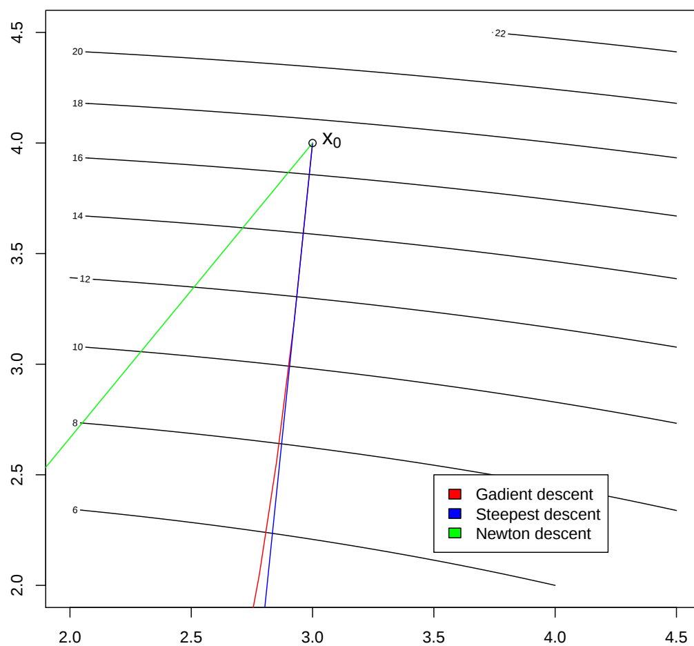
Figure 5.23: Zbliżenie ścieżek uzyskanych metodą Newtona i innych podobnych algorytmów
