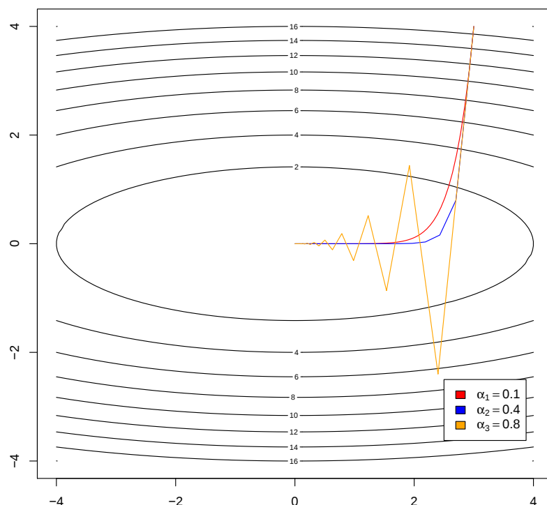
Figure 4.17: Wpływ learning rate na ścieżkę przebytą przez metodę gradientu prostego na funkcji f .
