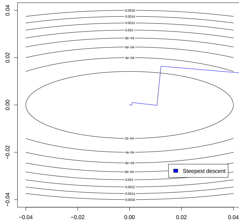
Figure 4.21: Zbliżenie ścieżki uzyskanej przez metodę najszybszego spadku na funkcji f w przestrzeni 2D
